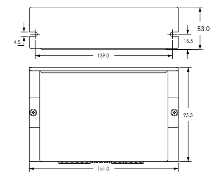
DMA860E
