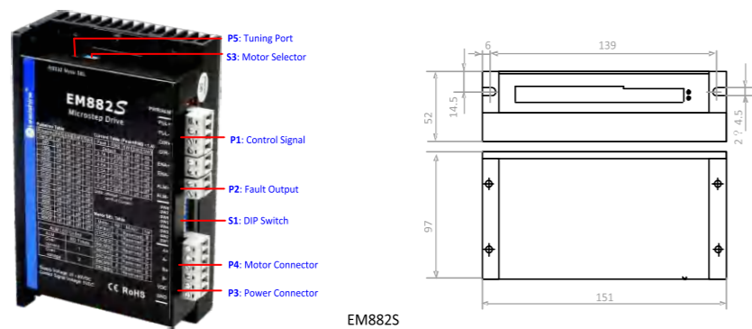
EM882S
