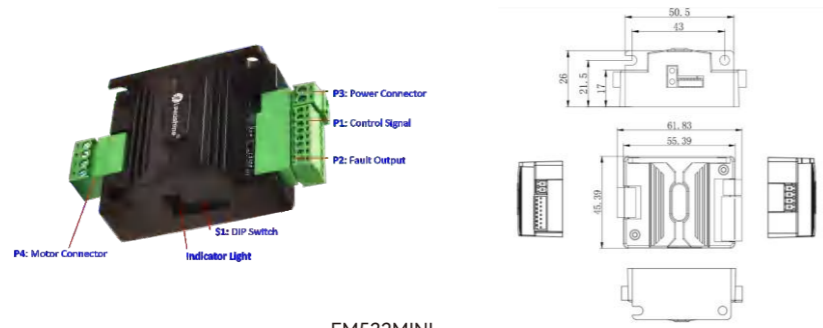
EM532MINI
