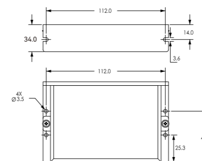
DM556E
