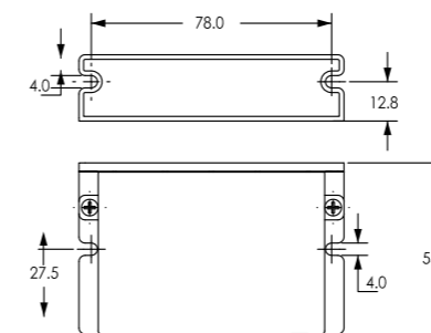
DM322E / DM332E
